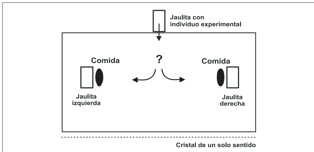
Figura 2. Diseño experimental utilizado para comprobar si los lúganos reconocen el babero negro de debajo del pico de sus compañeros como una verdadera señal de estatus social. Los diferentes pájaros experimentales se colocaban en la jaulita externa, y mediante un mecanismo accionado por el observador, se hacían pasar al interior de la jaula experimental. El experimento consistía en ver si el pájaro experimental prefería comer al lado del pájaro de mancha grande o con el de mancha pequeña, instalados en cada una de las jaulitas.
