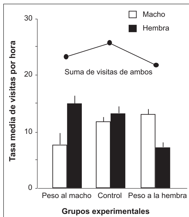
Figura 4. Tasa de visitas al nido por hora de observación en estorninos ( Sturnus vulgaris ), según tratamientos experimentales consistentes en colocar un sobrepeso a uno de los miembros de la pareja. El esfuerzo extra realizado por el otro miembro hace que la suma de las visitas de ambos no descienda en exceso, pero como se aprecia la compensación es sólo parcial. Redibujado de Clutton-Brock y Godfray (1991).
