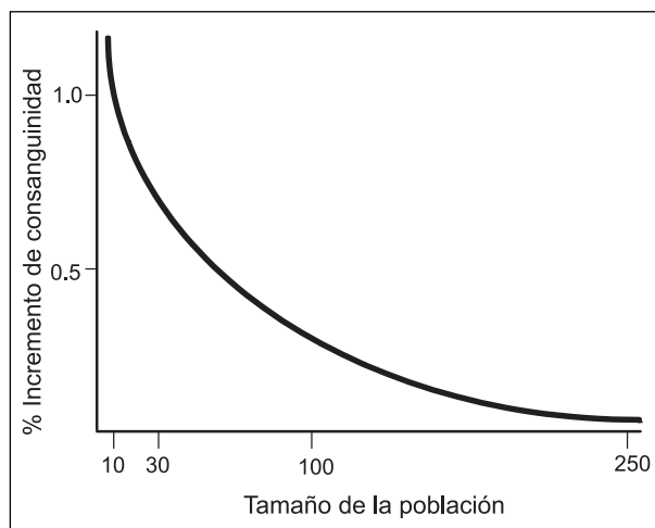
Figura 5. Relación entre el tamaño de la población y el aumento en el porcentaje de consanguinidad poblacional en cada generación, estimada para una población sexual panmíctica y con proporción de sexos 1:1.
