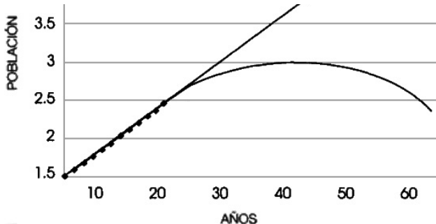
Figura 5. Nos fijamos en una escala más amplia. Otros modelos también encajan muy bien.
