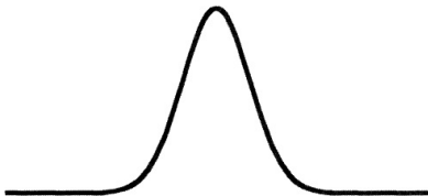
Figura 10. Una version mas abstracta: la curva de Platón. Un número infinito de lanzamientos.
