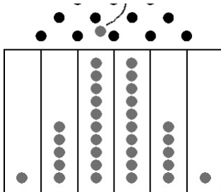
Figura 8. El quincix (simplificado): una máquina flipper. Soltemos las bolas de forma que, con cada golpe, caigan aleatoriamente a la derecha o a la izquierda. El resultado que la figura representa es el más probable, y se parece mucho a la curva de campana (también llamado distribución gaussiana). Cortesía de Alexander Taleb.
