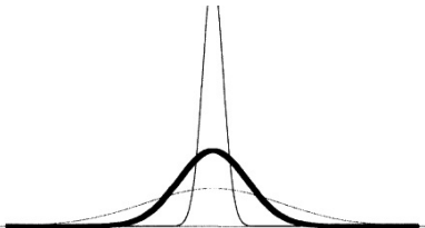
Figura 7. Cómo funciona la ley de los grandes números. En Mediocristán, a medida que nuestra muestra aumenta, el promedio observado se presentará cada vez con menos dispersión: como podemos ver, la distribución será cada vez más estrecha. Dicho en pocas palabras, así es como funciona (o se supone que funciona) toda la teoría estadística. La incertidumbre de Mediocristán se desvanece con el promedio. Esto ilustra la manida «ley de los grandes números».
