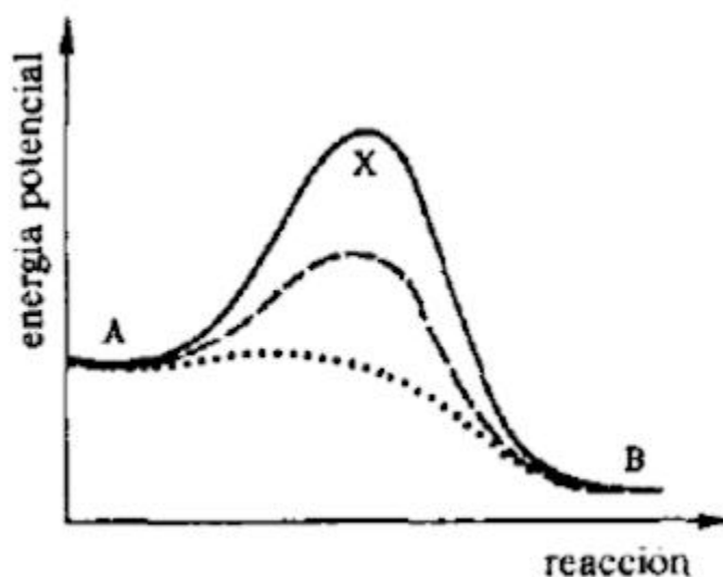
Fig. 1. Diagrama de la variación de la energía potencial de las moléculas en el curso de una reacción. A: estado estable inicial. B: estado estable final. X: estado intermedio, de energía potencial superior a la de los dos estados estables. Trazo continuo: reacción covalente. Trazo discontinuo: reacción covalente en presencia de un catalizador que disminuye la energía de activación. Trazo punteado: reacción no covalente.
