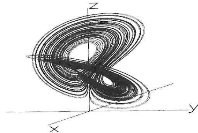
Figura 6-11 El atractor de Lorenz; de Mosekilde y otros (1994).
