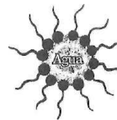
Figura 9-5 Forma básica de una gota «Micela».
