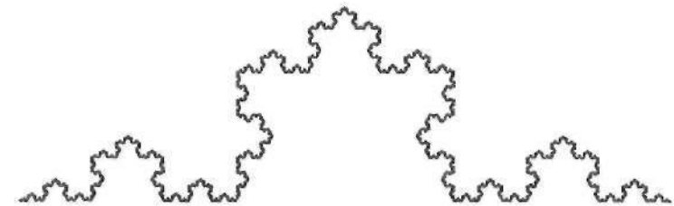
Figura 6-14 Representación de una línea de costa con la curva de Koch.
