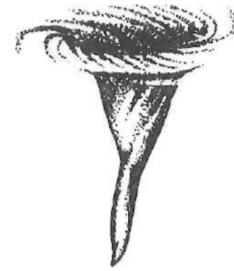
Figura 7-4 Embudo en forma de vórtice en el remolino de un desagüe.
